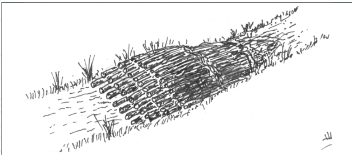
Obr. 148. Vrbo-olšový rošt – zához návodní strany filtru (vpravo) zeminou a kamenem. Záhozový materiál se získá odebráním z příkrých stěn strže. Prokládaná rovnanina z vrbových a olšových kmínků a větví. Kresba: Michal Bílý.
