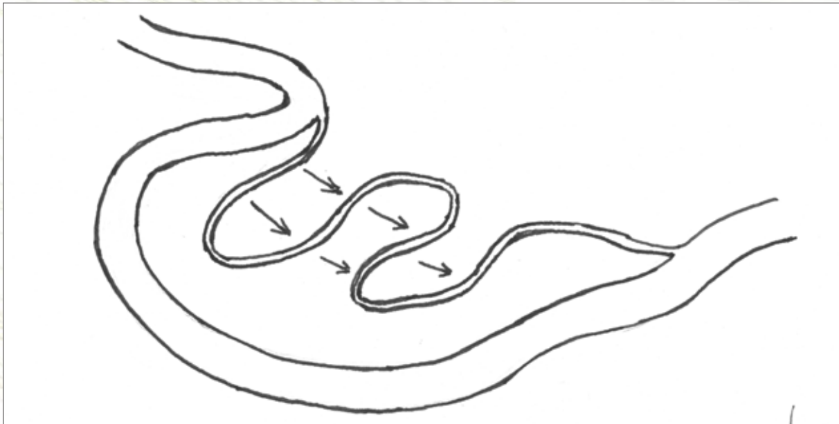
Obr. 137. Schéma ORP – meandrující luční koryto a jeho propojení s hlavním tokem. Šipky naznačují směr proudění podpovrchové vody rhizosférou (prokořeněnou zónou luční vegetace v průlincitěm štěrkovém základu) napříč meandry. Kresba: Michal Bílý.
